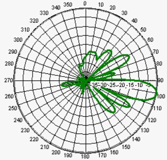
Freq: 850 MHz, Tilt: 10
