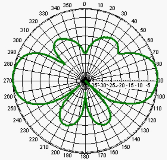
Freq: 903 MHz, Tilt: 0
