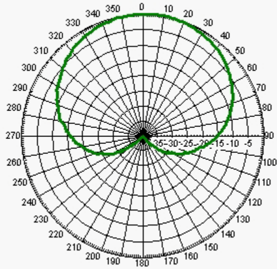
Freq: 835 MHz, Tilt: 6
